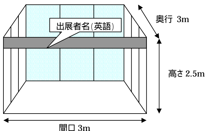
< 小間仕様図 >
